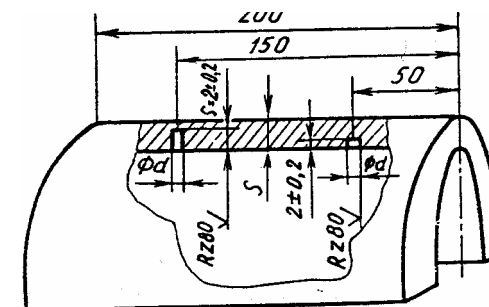
Неуказанные предельные отклонения размеров:
